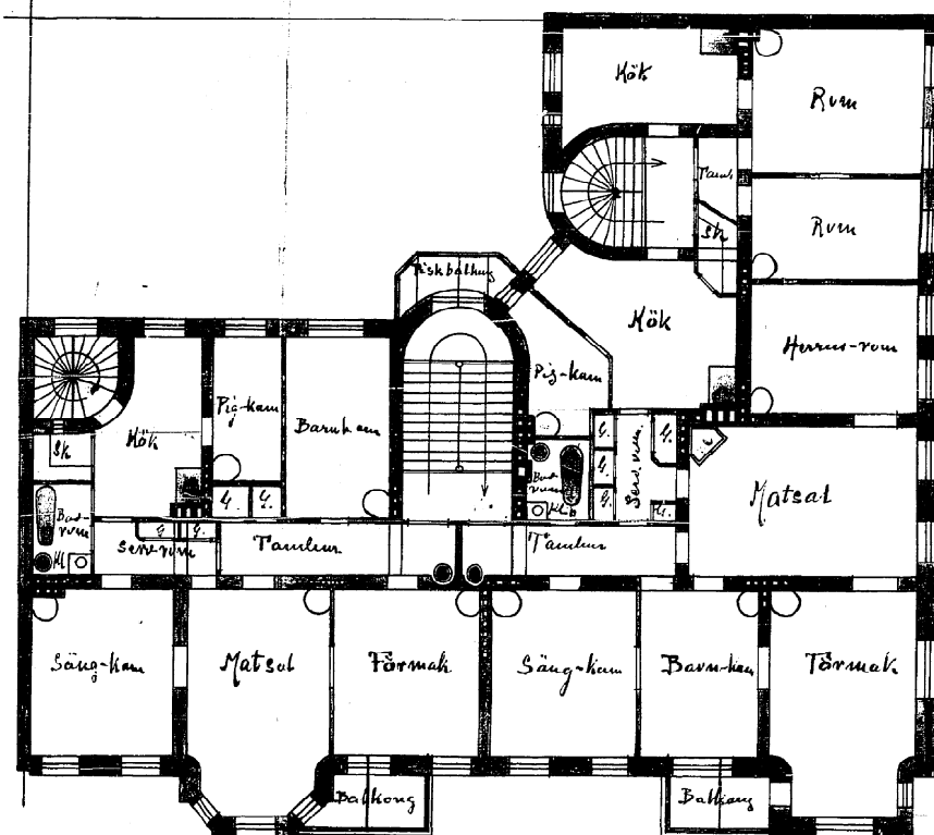
Plan af 4 de Vån.
