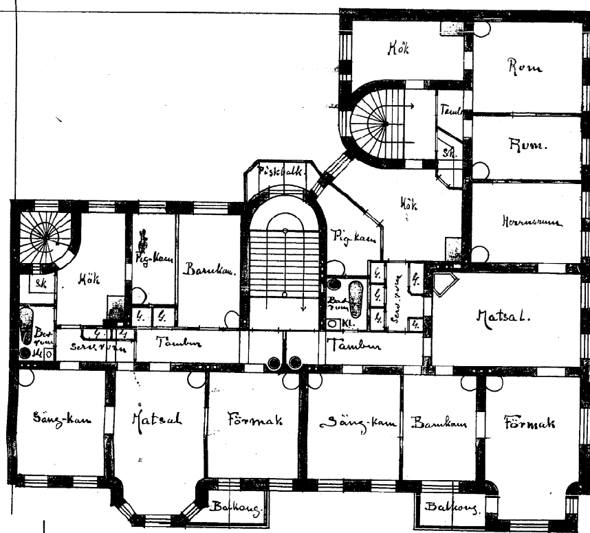
Plan af 2 de Vån.
